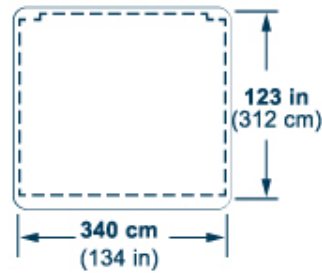
Side cargo door (STA 1850)
